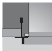
Instalace do rástrového podhledu zeshora
