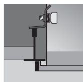
Instalace do rástrového podhledu zezdola
